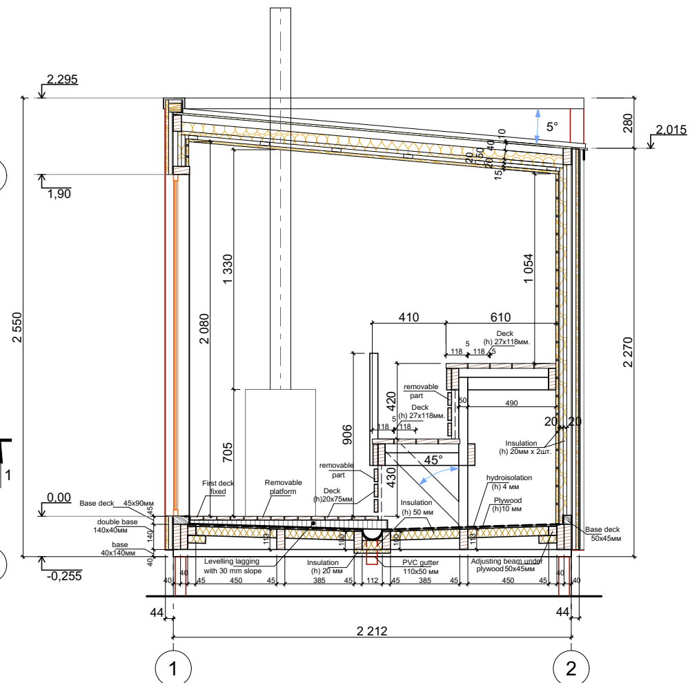
Slit 1-1.
